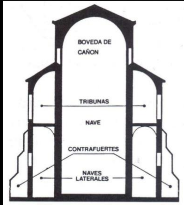
Alzado románico
